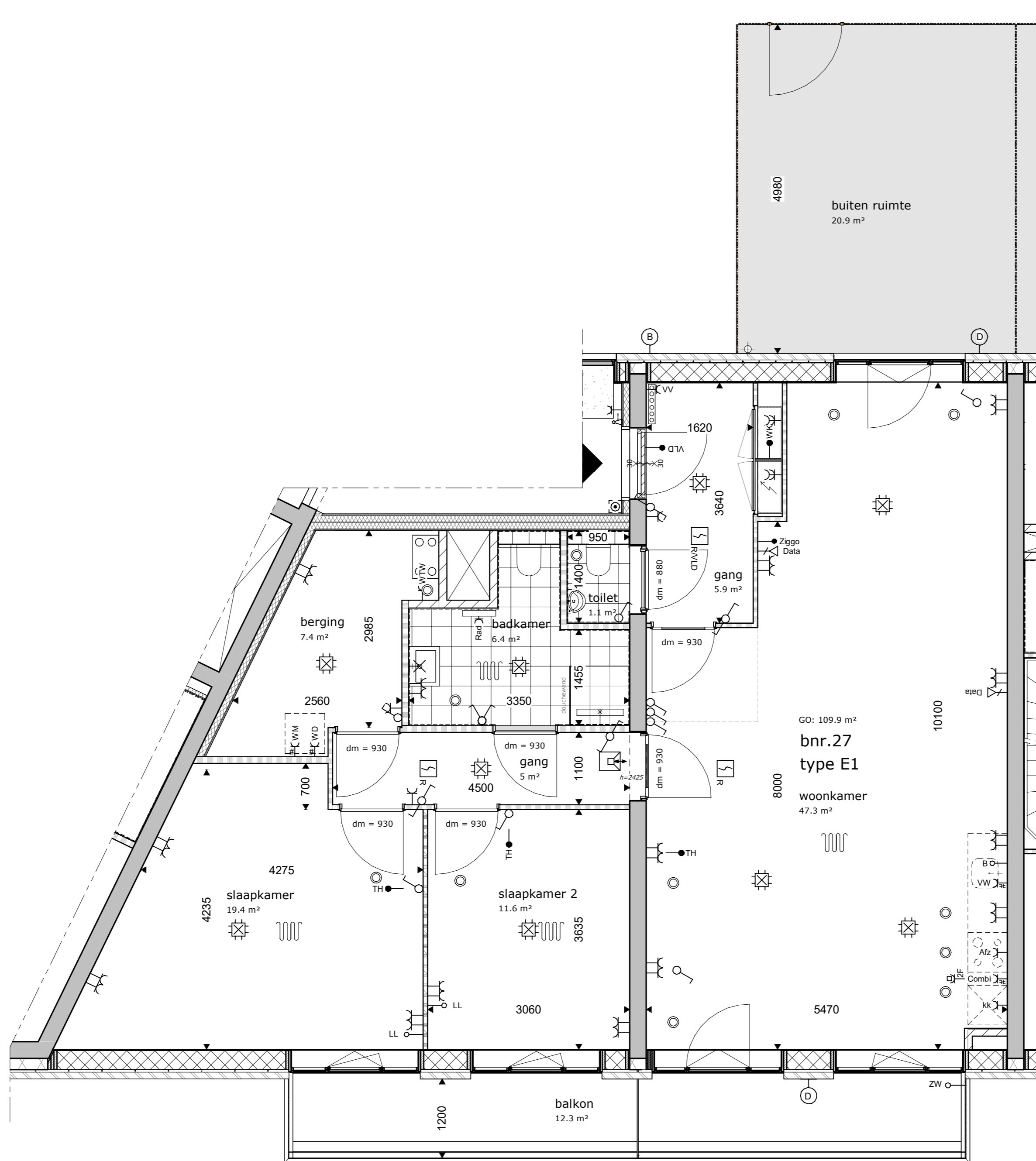
eerste verdieping type E1
