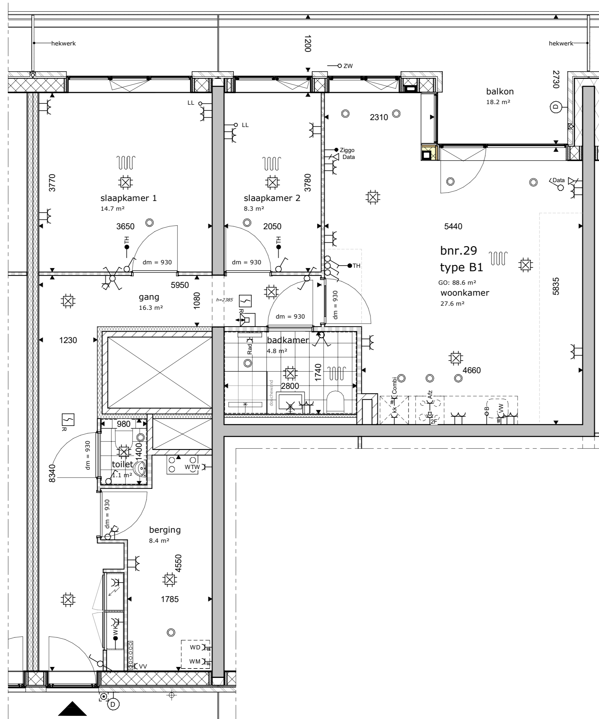
tweede verdieping type B1
