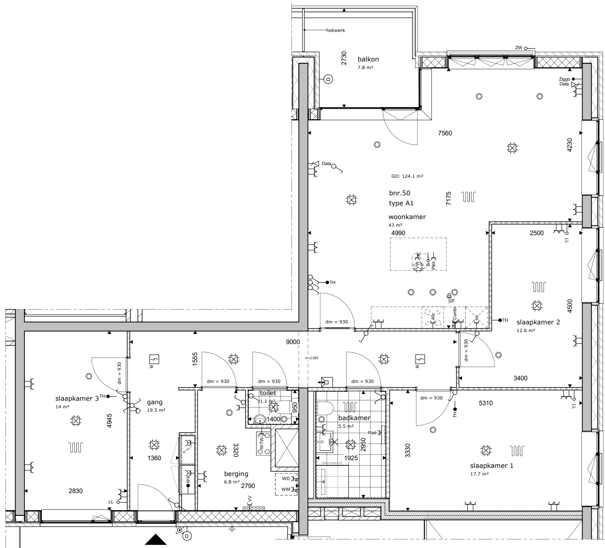
vierde verdieping type A1
