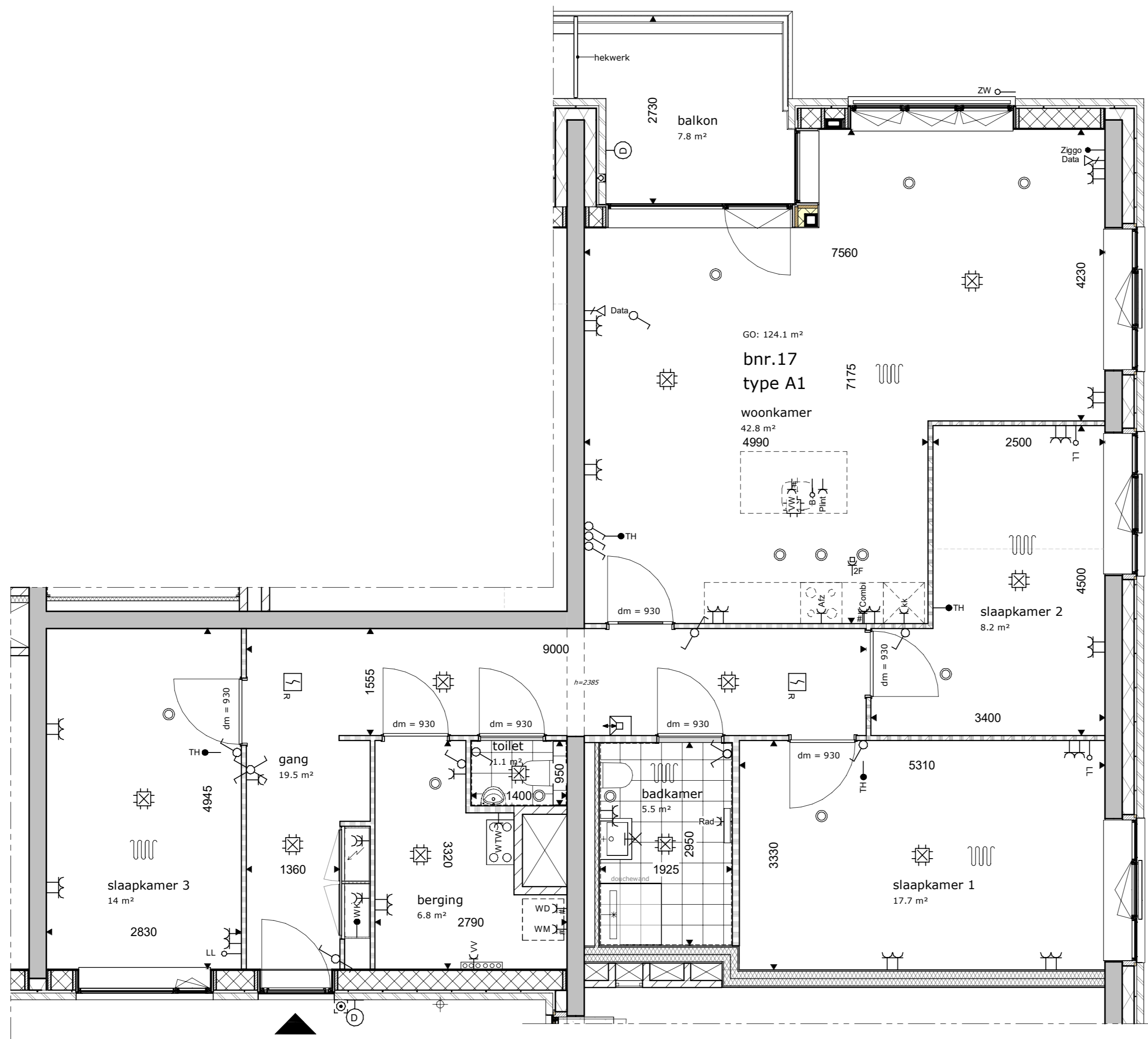
eerste verdieping type A1
