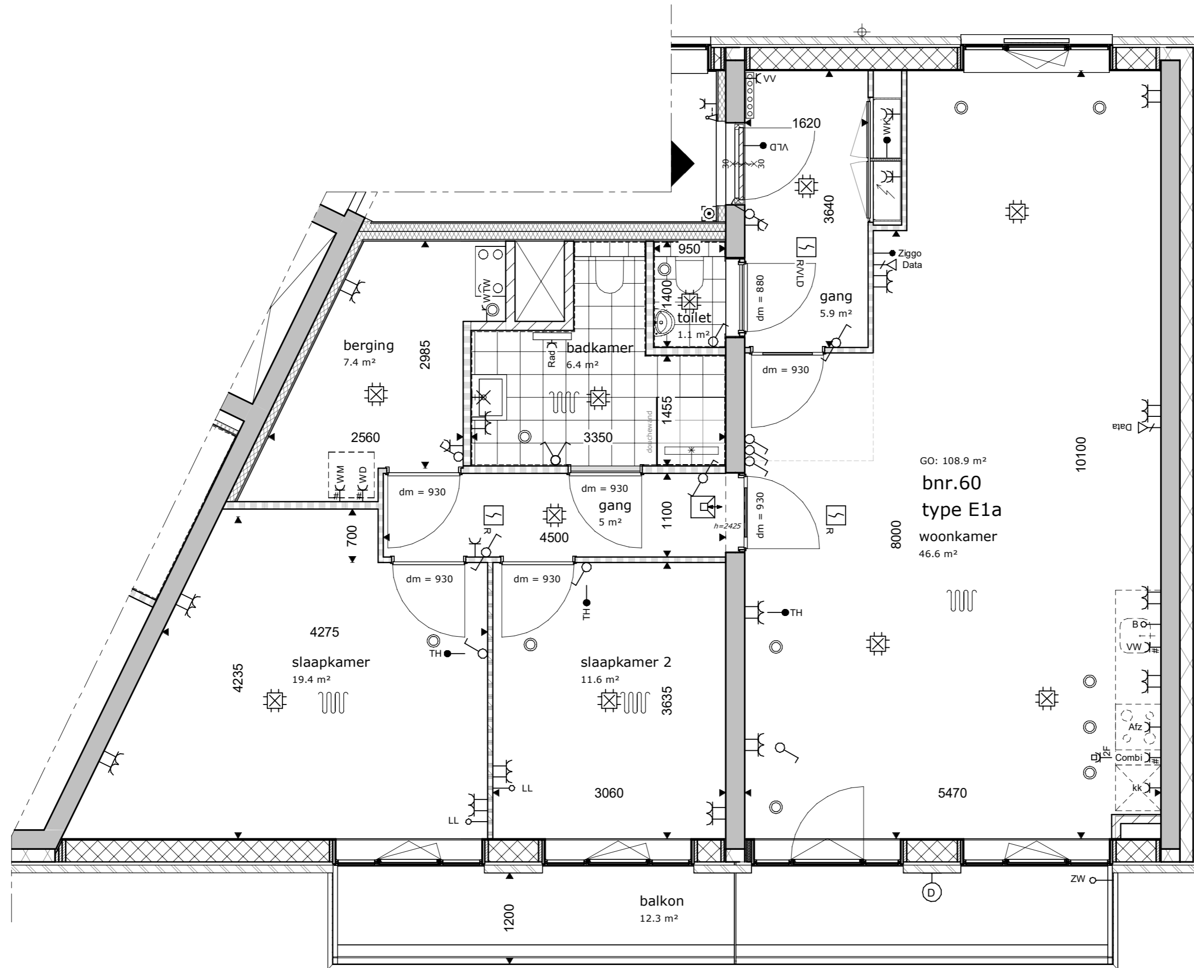
vierde verdieping type E1a
