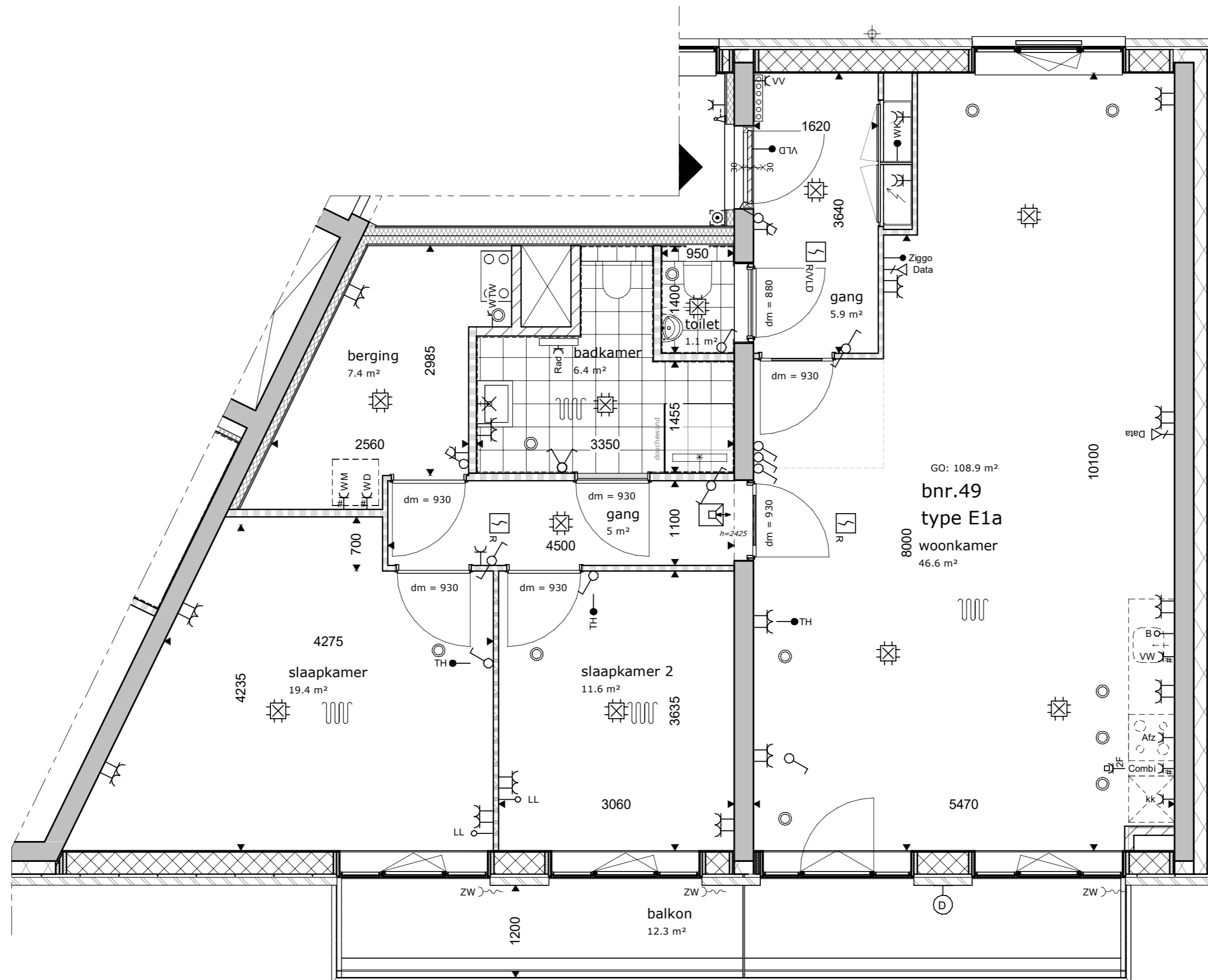
derde verdieping type E1a
