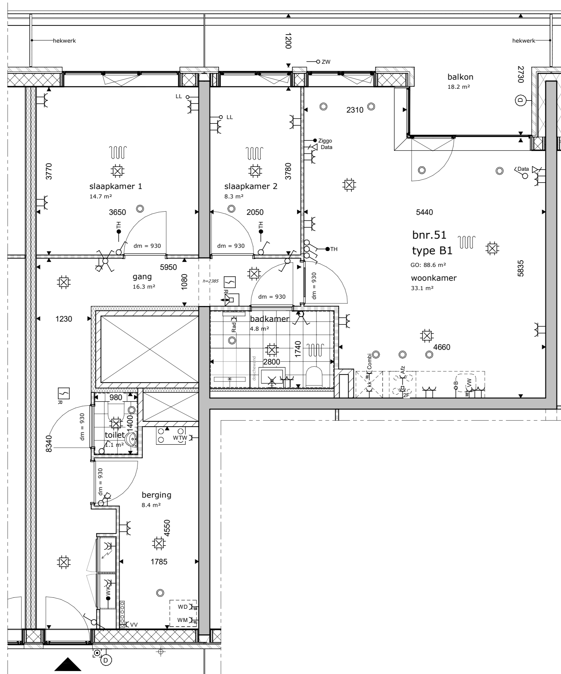
vierde verdieping type B1
