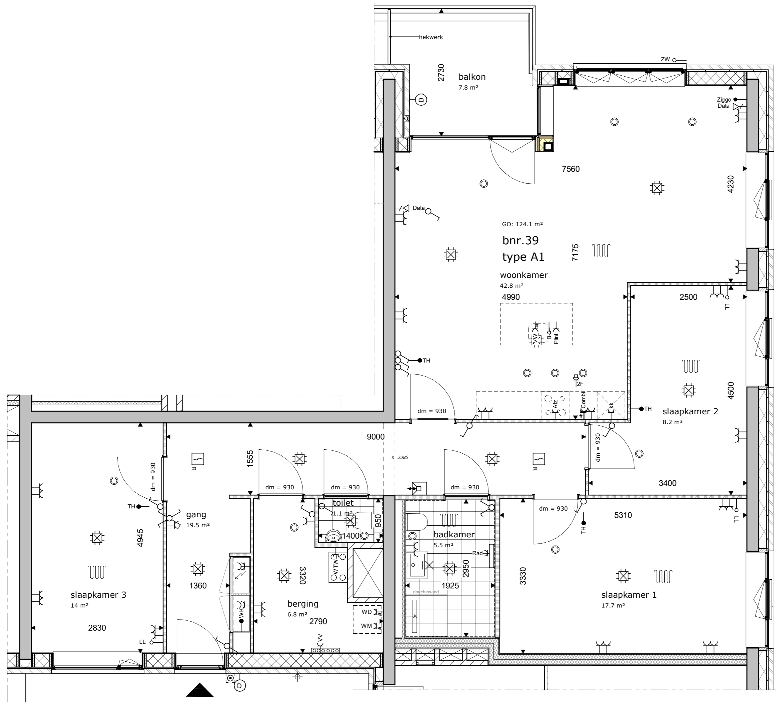
derde verdieping type A1
