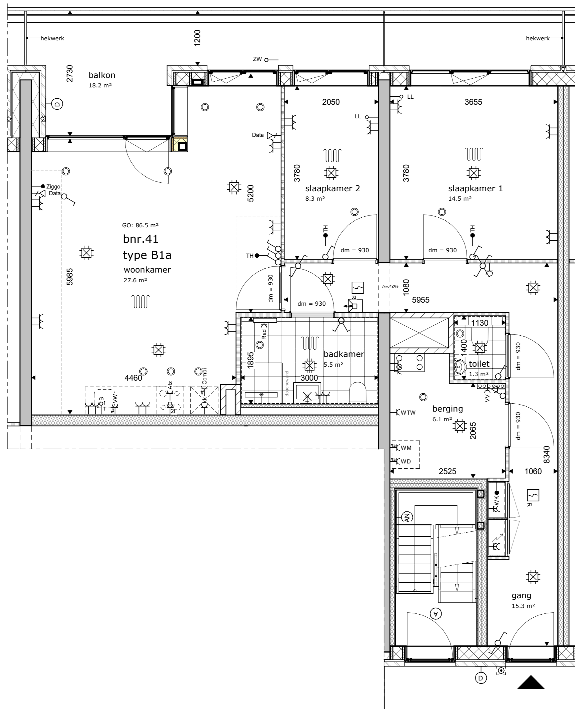
derde verdieping type B1a
