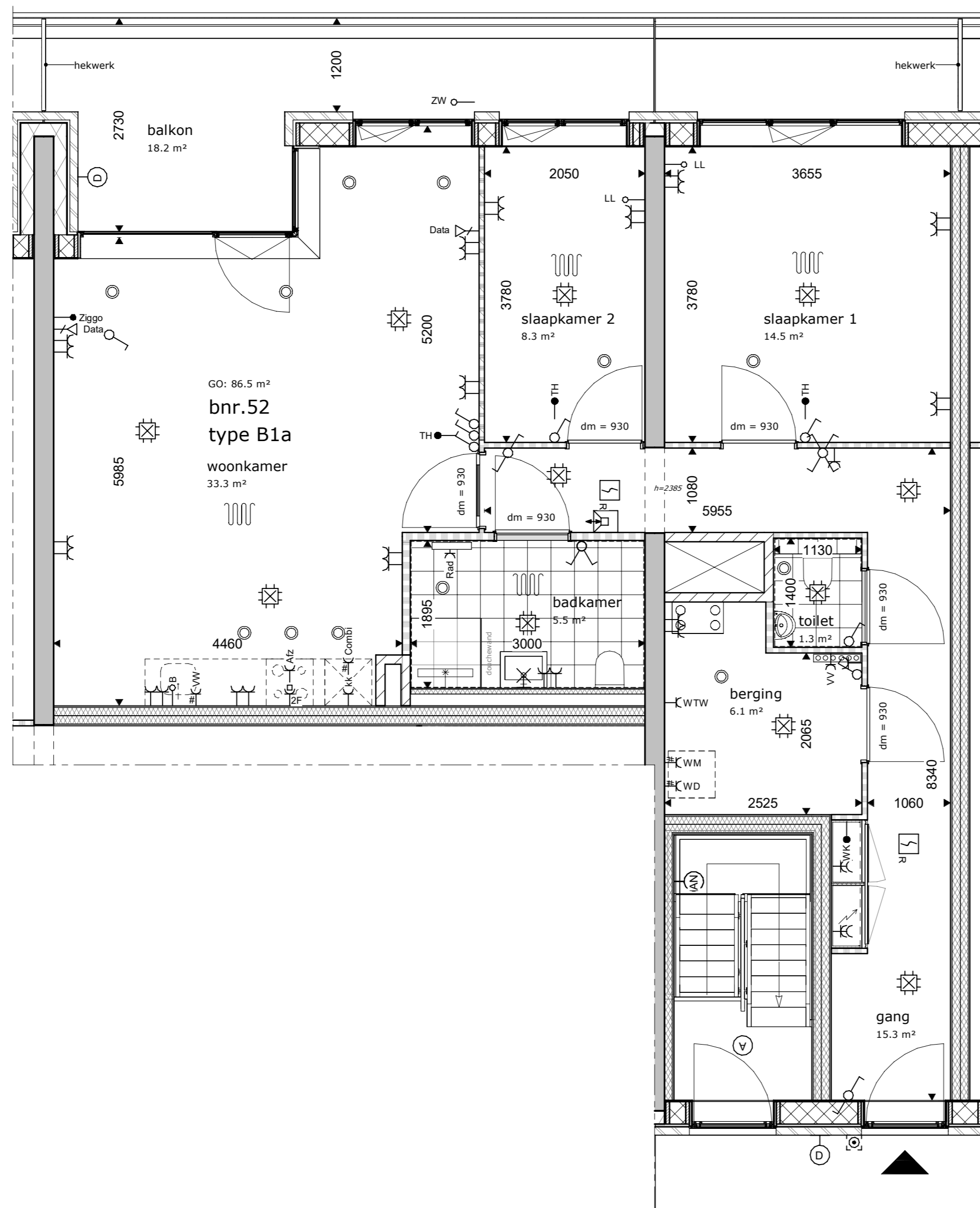
vierde verdieping type B1a
