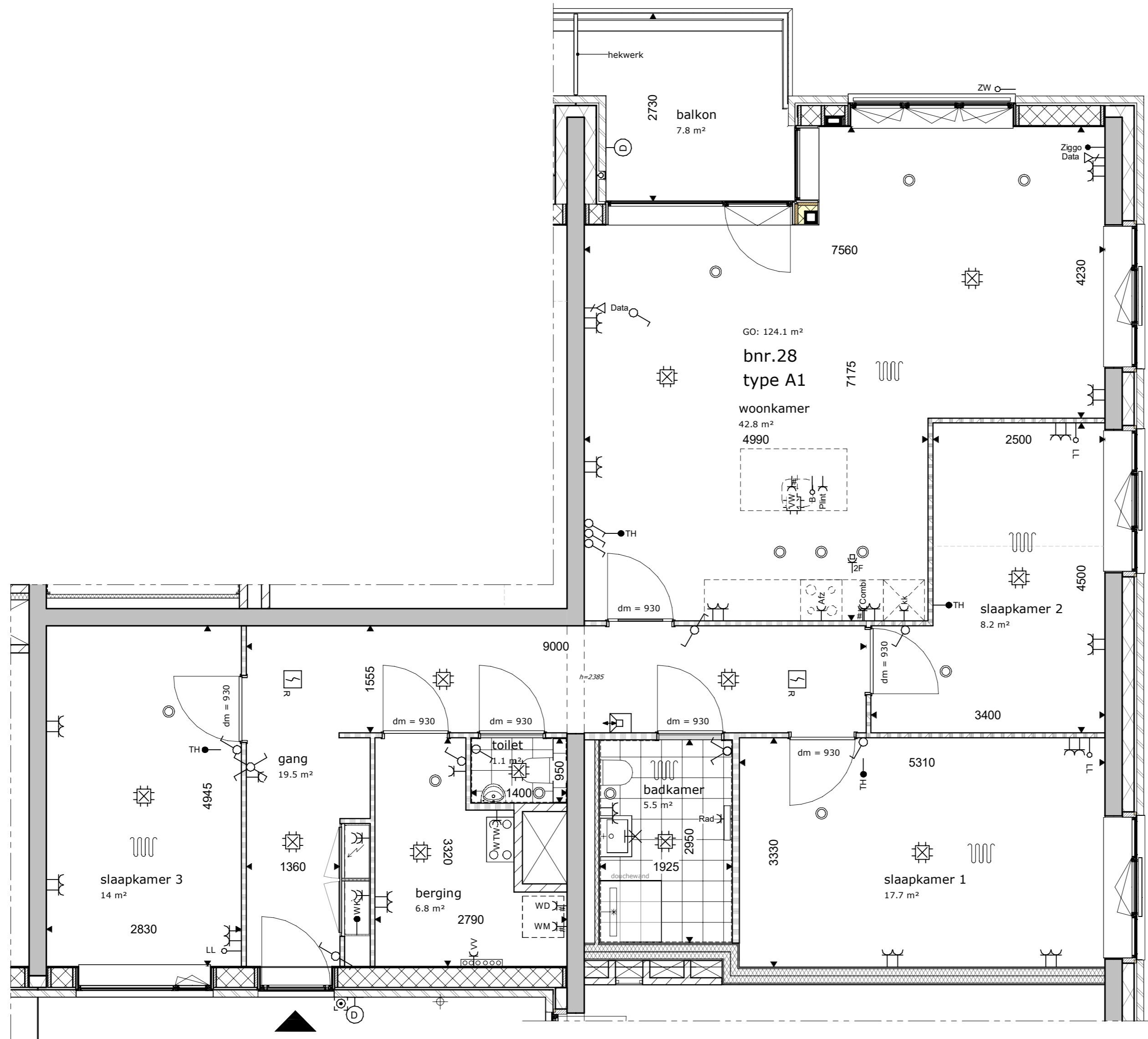
tweede verdieping type A1
