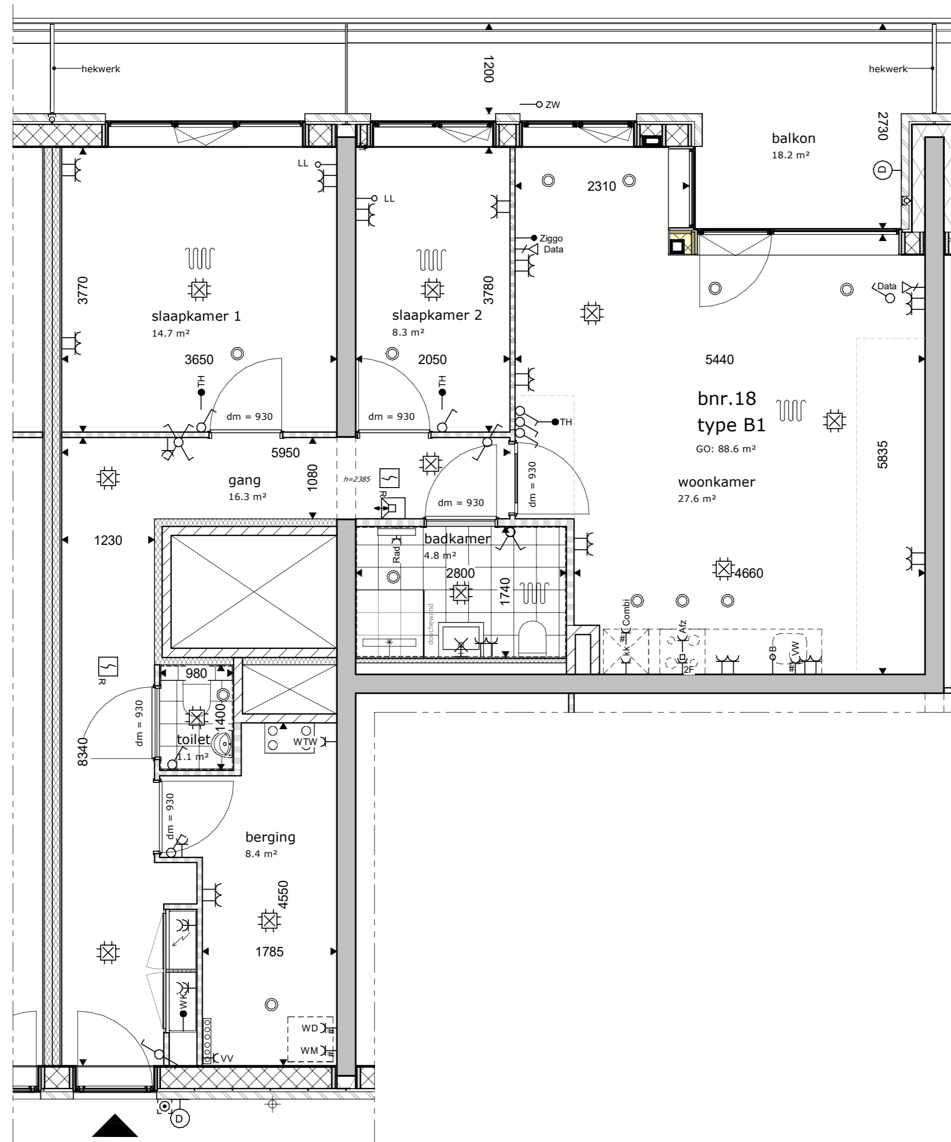
eerste verdieping type B1
