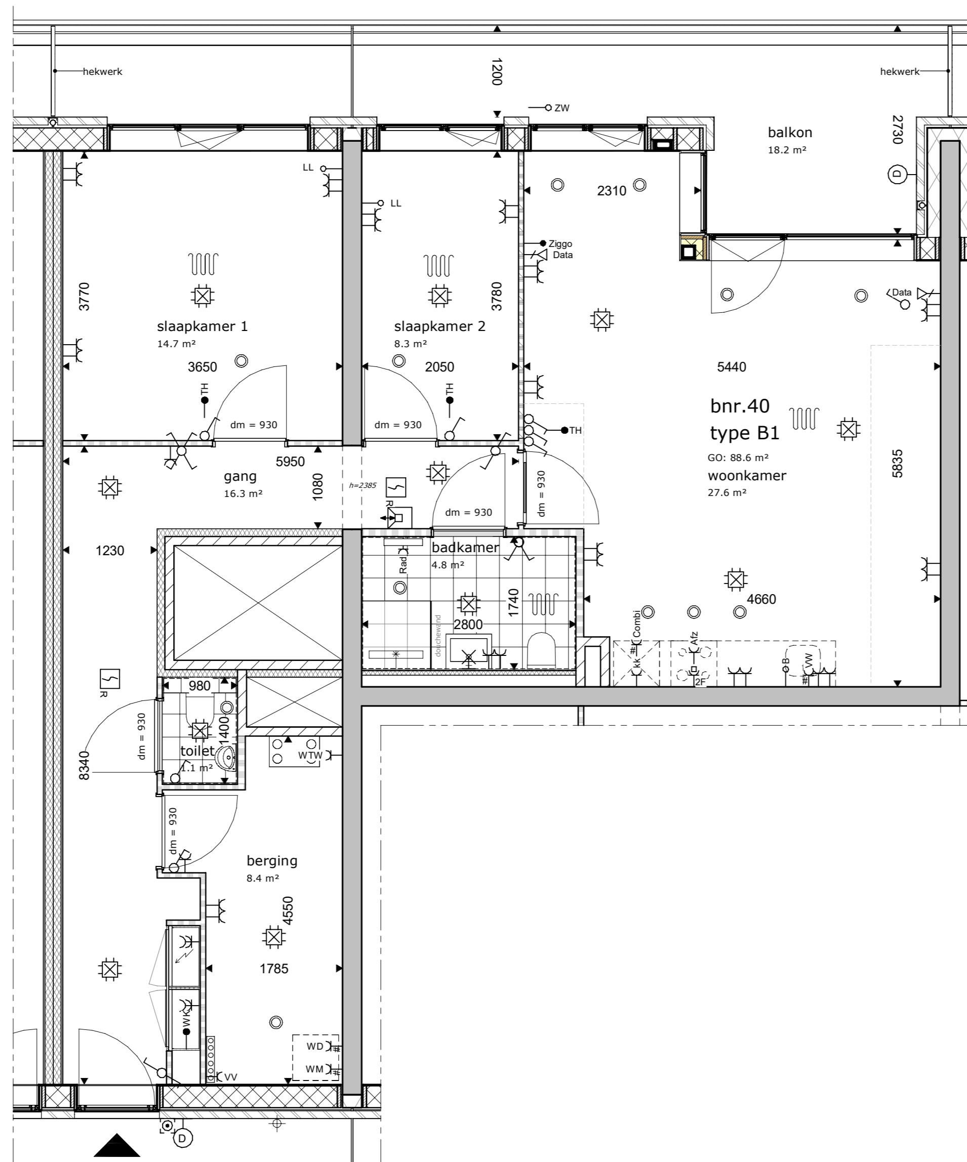
derde verdieping type B1
